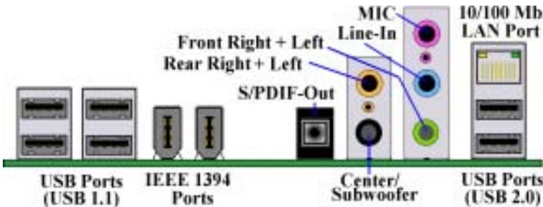
圖 2-9. AT7 背面面板的連接埠
