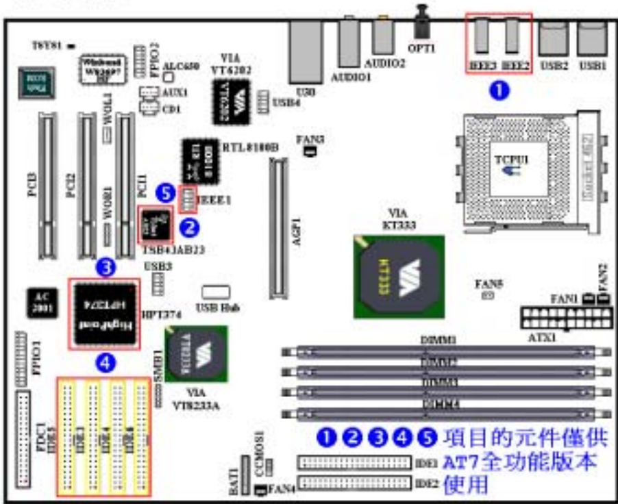
圖 1-1. AT7/AT7E 主機板重要元件位置圖
