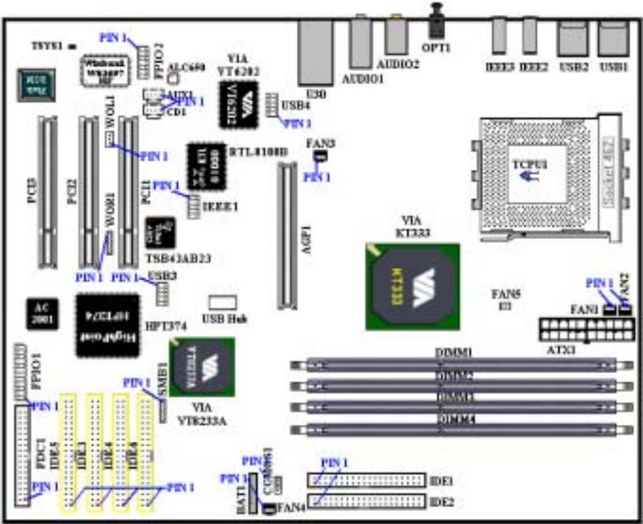
圖 2-7. AT7 主機板的所有連接埠和接頭
