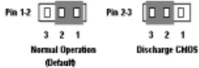
圖 2-8. CCMOS1 插梢的設定
