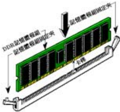
圖 2-6. DDR 記憶體模組的安裝 仍要繼續做其它的動作均可。
