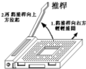
圖2-3. 將Socket A的推桿拉起
