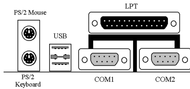
Figure 2-11. Connecteurs d'entrées/sorties de votre BE6.
