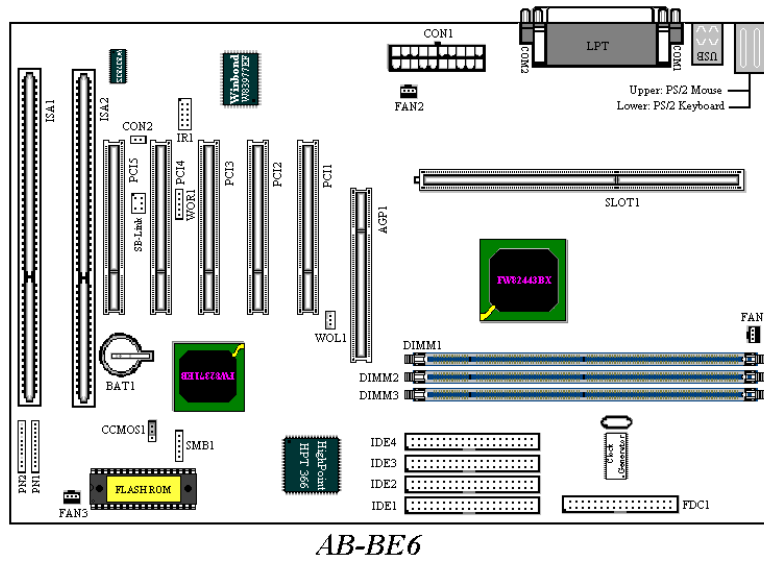
Figure 1-2 Emplacement des composants de la carte mère
