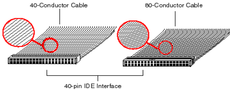
Figure 2-8. Comparaison câble Ultra-ATA/33 et câble Ultra-ATA/66
