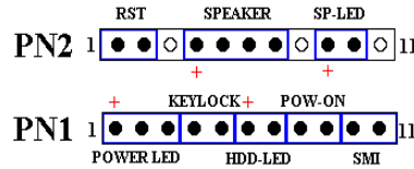
Figure 2-7. Définitions des pins du PN1 et PN2
