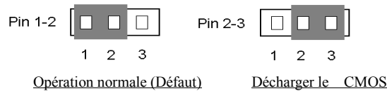
Figure 2-6. Paramètre du CCMOS1
