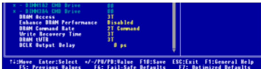
図 3-5B. DRAM クロック/ドライブコントロールの下部画面
