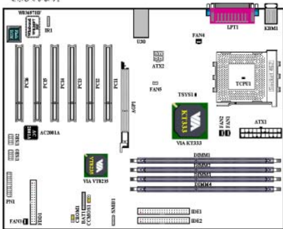
図 1-1. KD7-E のコンポーネントの位置
