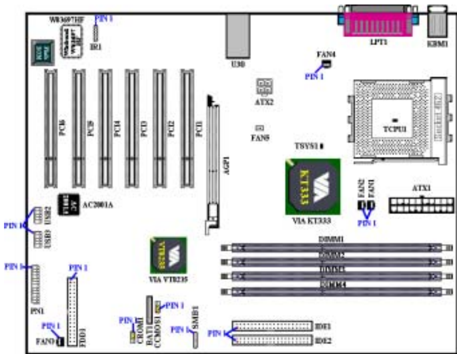
図 2-7. KD7-E のコネクタとヘッダー
