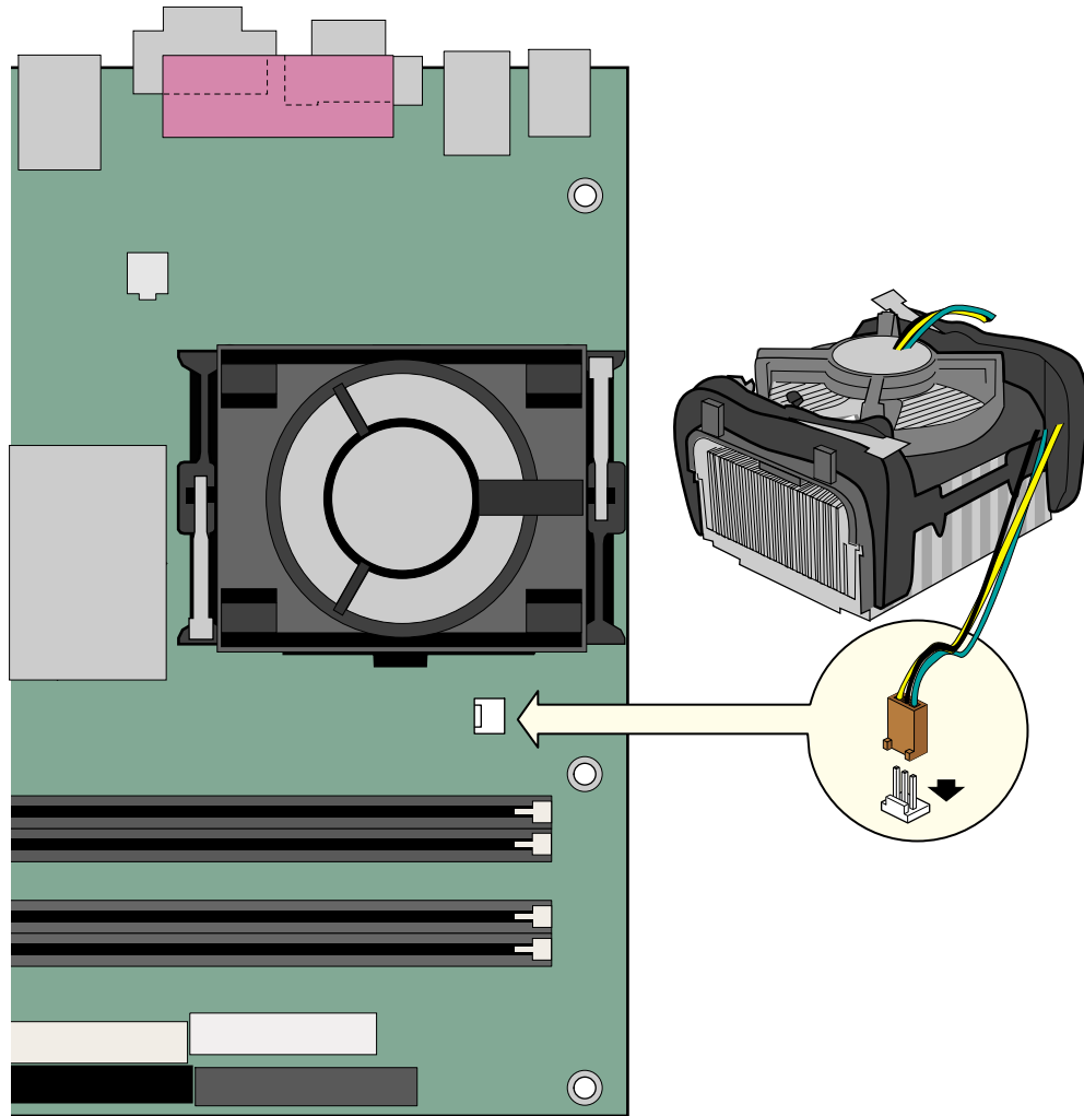
그림 6. 프로세서 팬 커넥터에 프로세서 팬 방열기 케이블 연결하기
