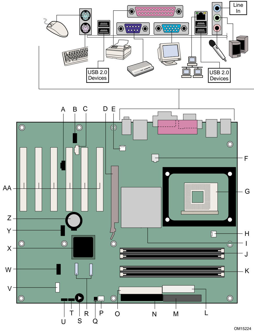
그림 1. 데스크톱 보드 D865GBF 부품
