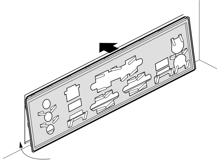
그림 3. I/O 실드 설치하기
