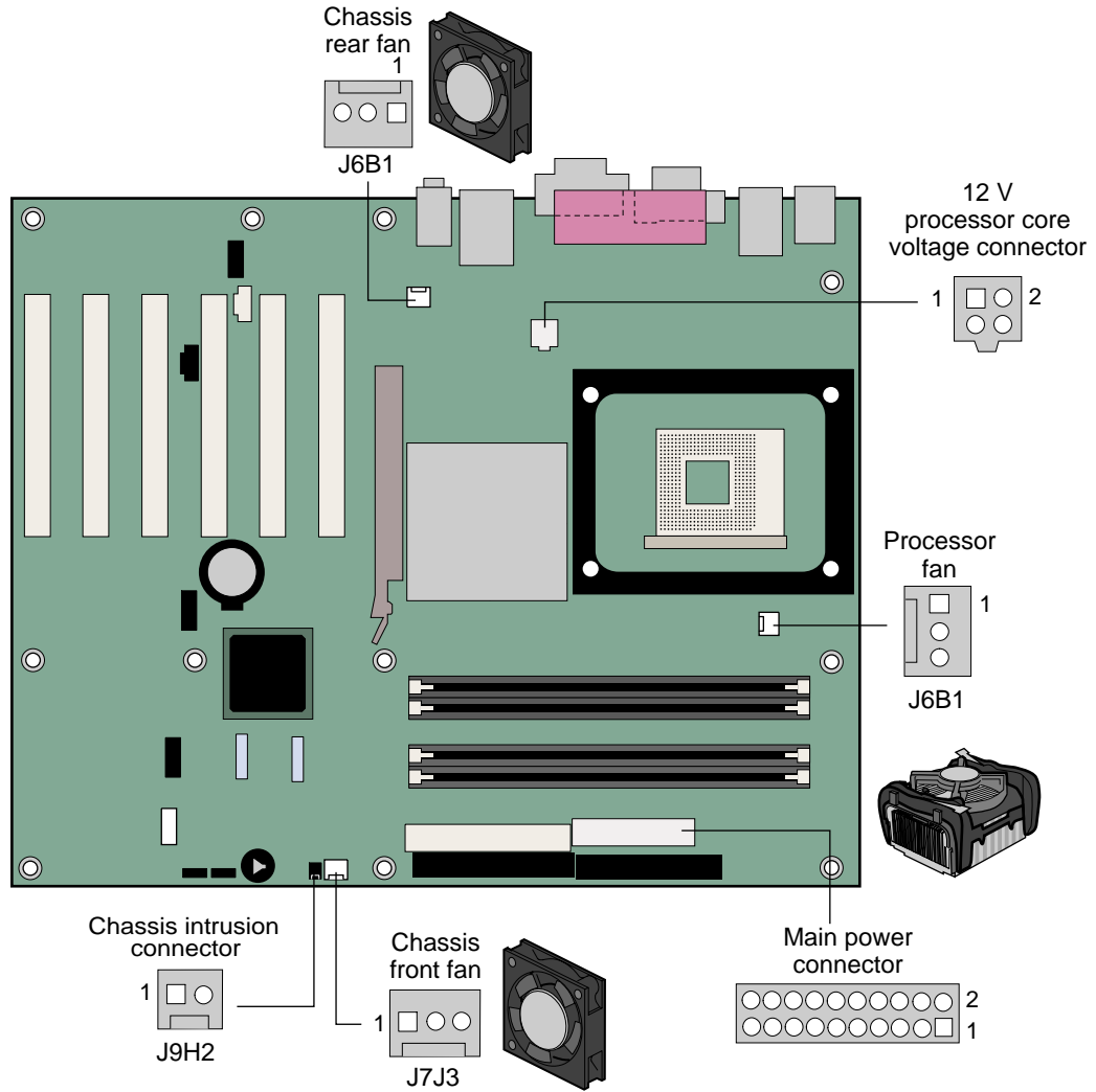
그림 15. 하드웨어 제어 커넥터 및 전원 커넥터의 위치
