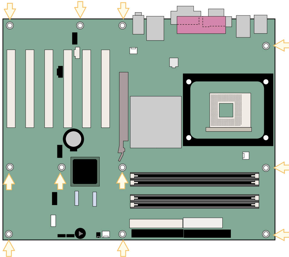
그림 4. 데스크톱 보드 설치 나사 구멍의 위치
