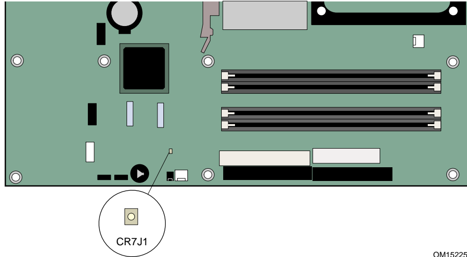
그림 2. 대기 전원 표시등의 위치
