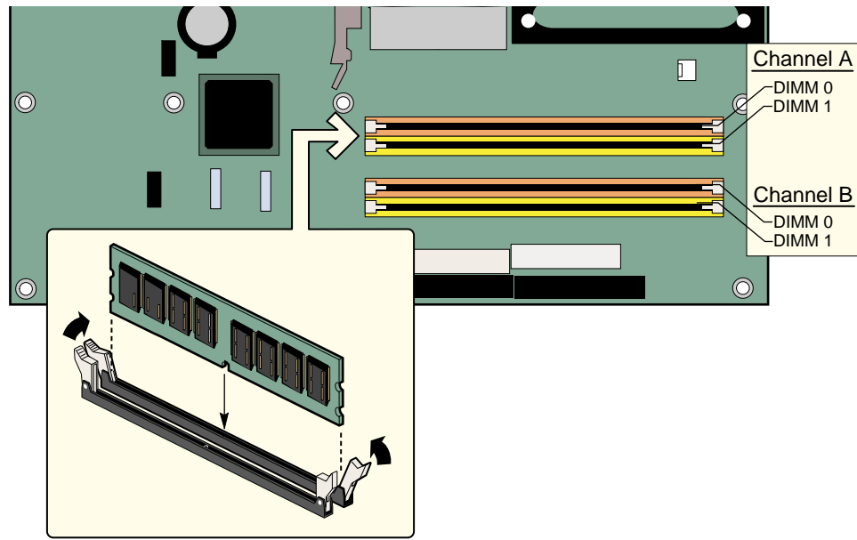
그림 7. 메모리 모듈 설치하기
