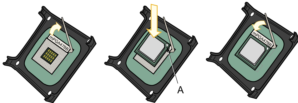
그림 5. 프로세서 설치하기
