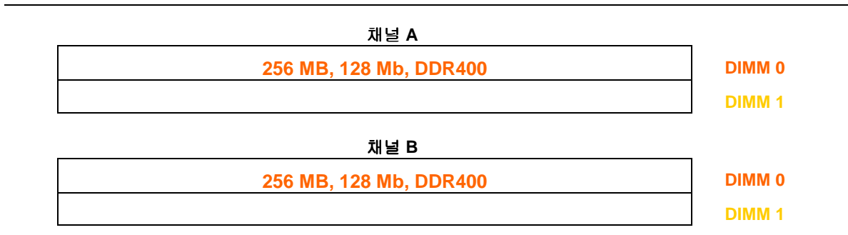
그림 8. 2 개의 DIMM 을 사용한 듀얼 구성의 예
