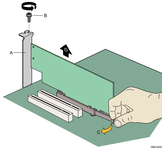
그림 10. AGP 카드 제거하기
