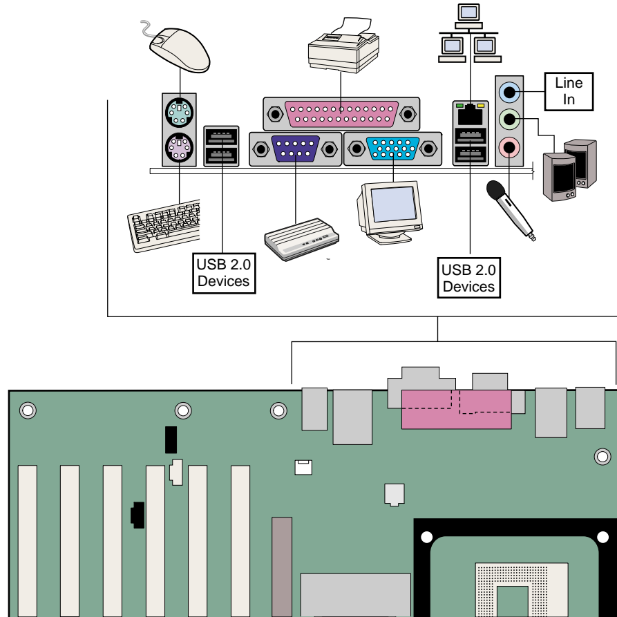
그림 18. 후면 패널 커넥터
