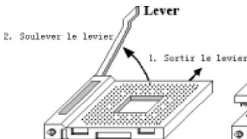
Schema 2-3. Socle A et son levier ouvert
