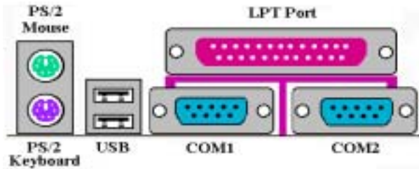
Figure 2-11. Connecteurs du panneau arrière de la KR7A/KR7A-RAID
