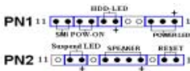
Figure 2-9. Définitions des pins des PN1 et PN2
