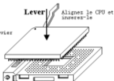
Schema 2-4. Installer le CPU dans le Socle A
