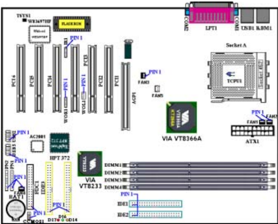
Figure 2-7. Tous les connecteurs et Switches de la KR7A/KR7A-RAID
