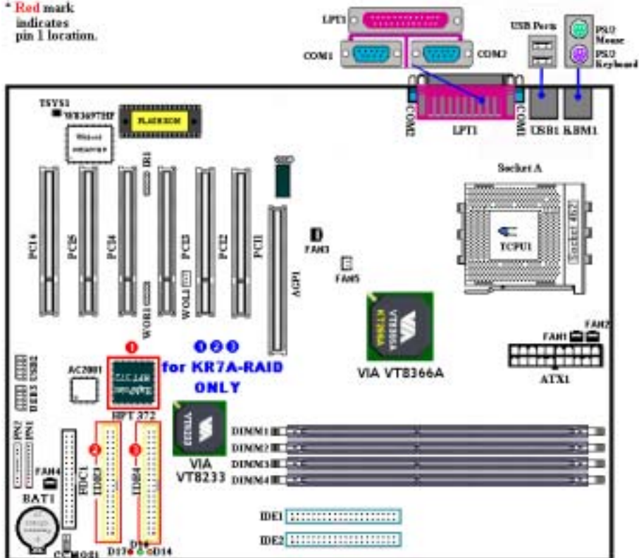
Figure 1-1. Emplacement des composants sur la KR7A/KR7A-RAID
