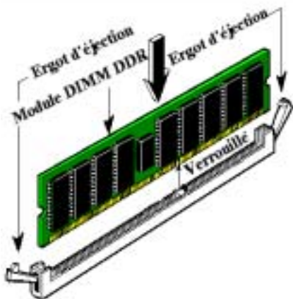
Figure 2-6. Installation du module mémoire DDR
