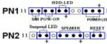
Illustration 2-9. Définitions des pins des PN1 et PN2
