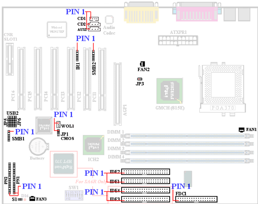
図 2-7. SA6/SA6R のコネクタとヘッダ
