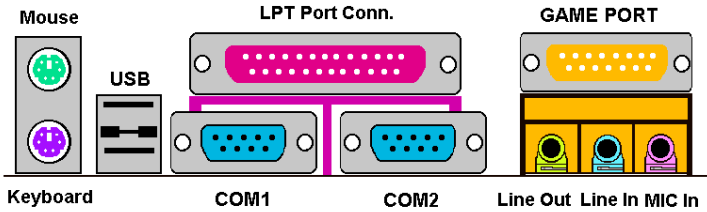
図 2-11. SA6/SA6R のバックパネルのコネクタ
