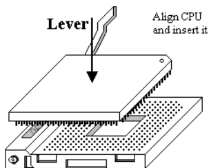
図 2-4. Socket 370 プロセッサのインストール
