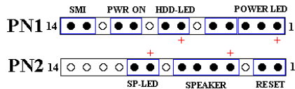
図 2-9. PN1 と PN2 の設定
