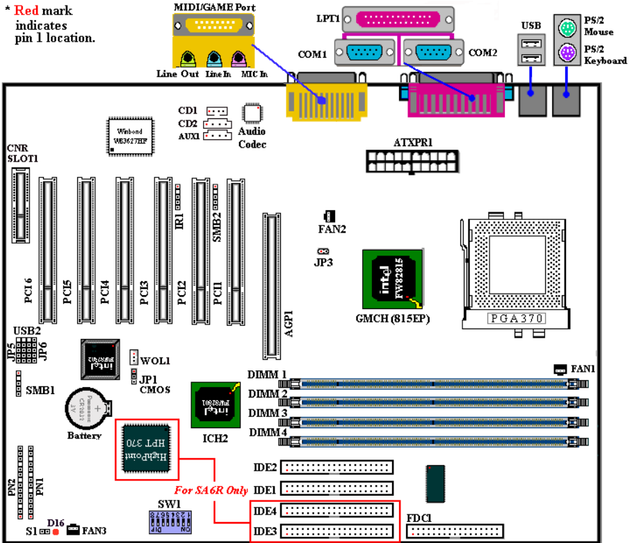
Abb. 1-1. SA6/SA6R Anordnung der Komponenten
