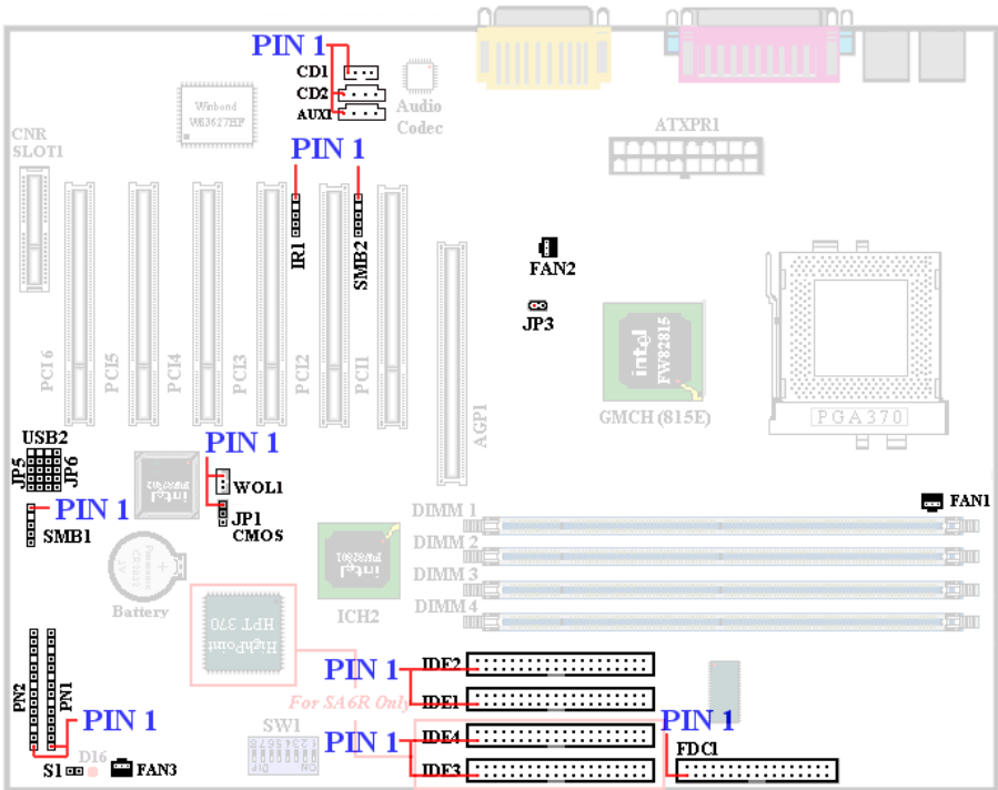
Abb. 2-7. Die Anschlüsse und Headers des SA6/SA6R
