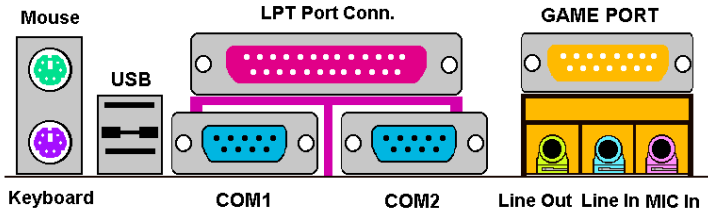
Abb. 2-11. Anschlüsse auf der Rückseite des SA6/SA6R
