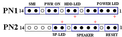
Abb. 2-9. Definition der Stifte PN1 und PN2
