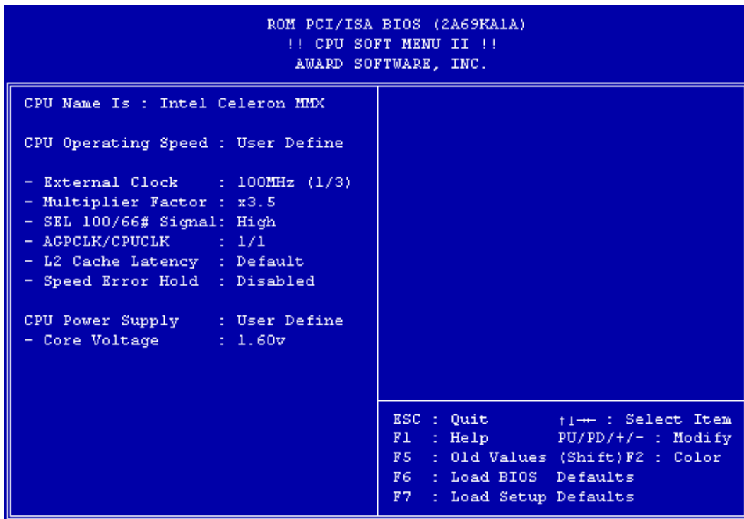
圖 3-2 CPU SOFT MENU™ II
