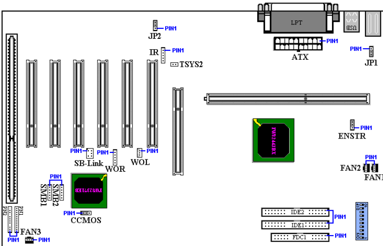
Figure 2-5. Connecteurs et prises de la BF6
