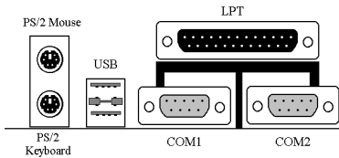
Figure 2-8. Connecteurs d’entrées/sorties de votre BF6.
