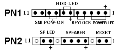
圖 2-7. PN1 以及 PN2 各腳 PIN 間之功能名稱
