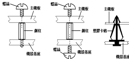
圖 2-2. 固定主機板至機殼的幾種方法
