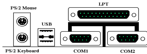
圖 2-11. BE6-II 背板之連接器
