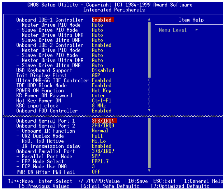
圖 3-7. 整合週邊設定選單畫面
