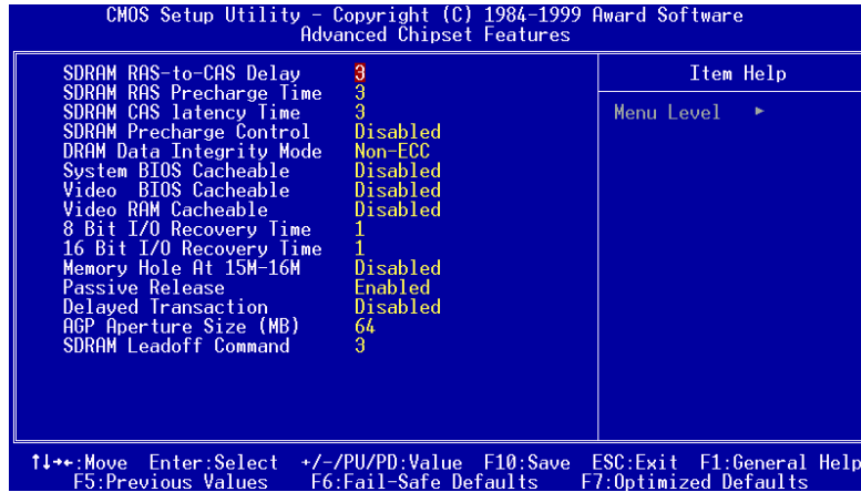
圖 3-6. 晶片組進階功能參數設定選單畫面
