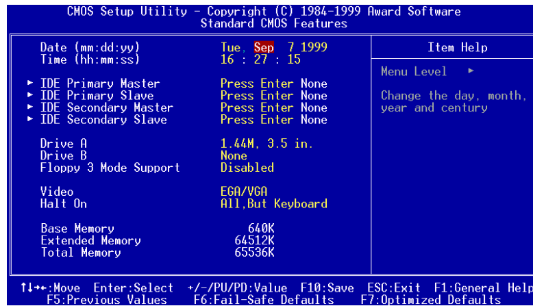
圖 3-3. Standard CMOS 設定選單畫面
