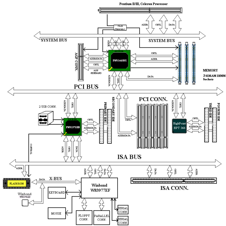
圖 1-2. BE6-II 主機板系統方塊圖
