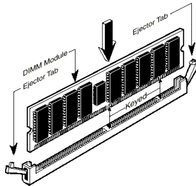
圖 2-4. 記憶體模組的安裝
