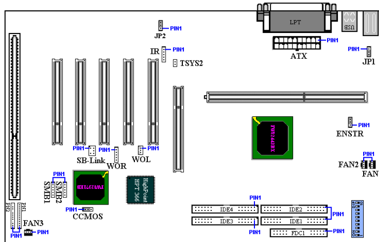
圖 2-5. BE6-II 所有有用到的連接器及連接頭位置圖
