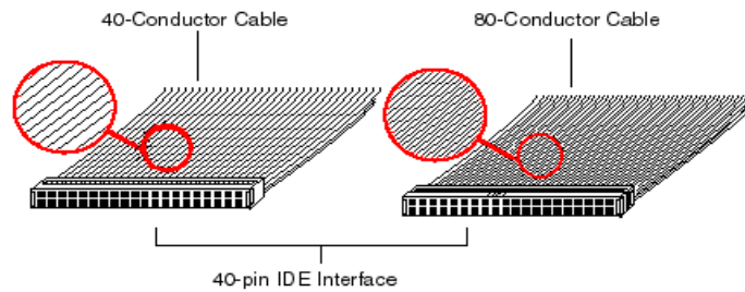
圖 2-8: Ultra ATA/33 與 Ultra ATA/66 排線之差異
