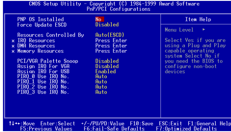
圖 3-9. PnP/PCI 組態設定畫面
