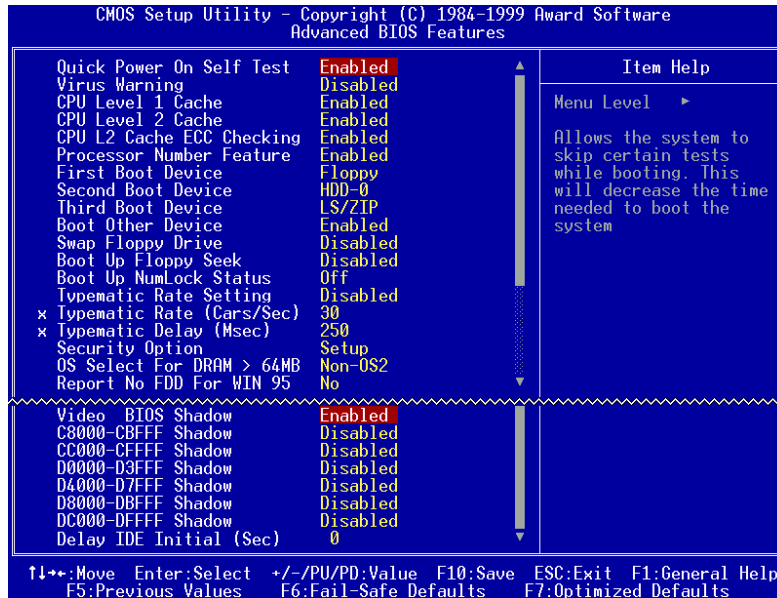
圖 3-5. BIOS 進階功能設定選單之畫面
