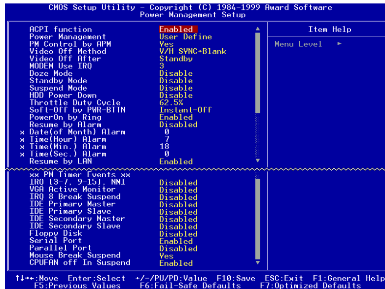
圖 3-8. 電源管理模式設定選單之畫面
