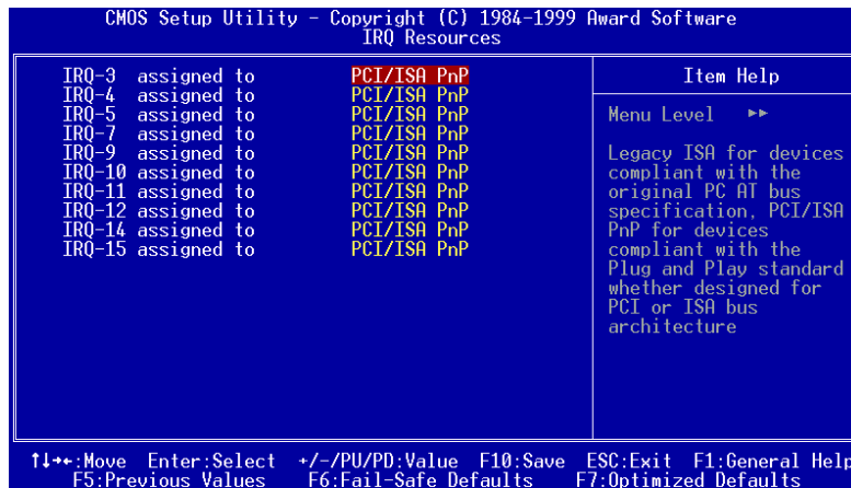
圖 3-10. PnP/PCI 組態 - IRQ 資源設定畫面
