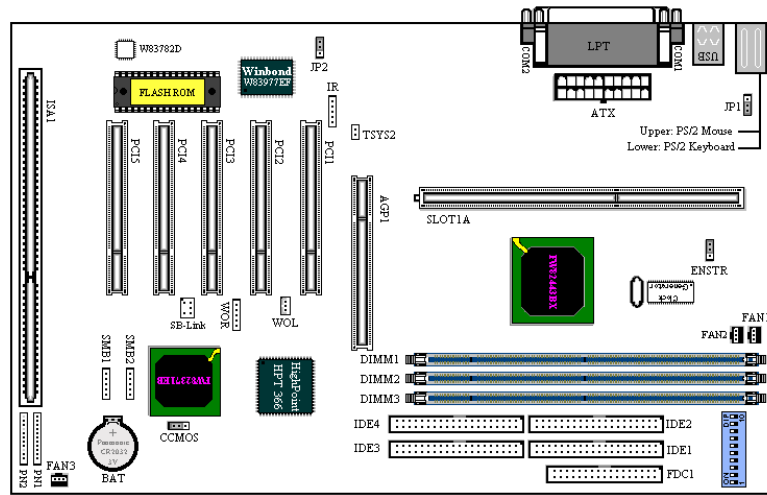
圖 1-1. BE6-II 主機板零件位置圖
