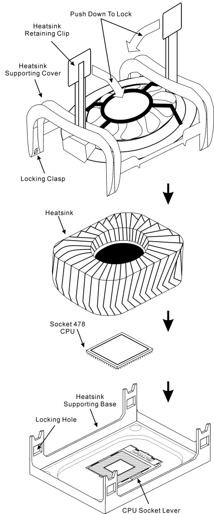
図 2-3. P4 ソケット 478 CPU およびそのヒートシンクをサポート台に取り付ける。
