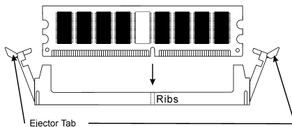
図 2-4. メモリモジュールの取り付け
